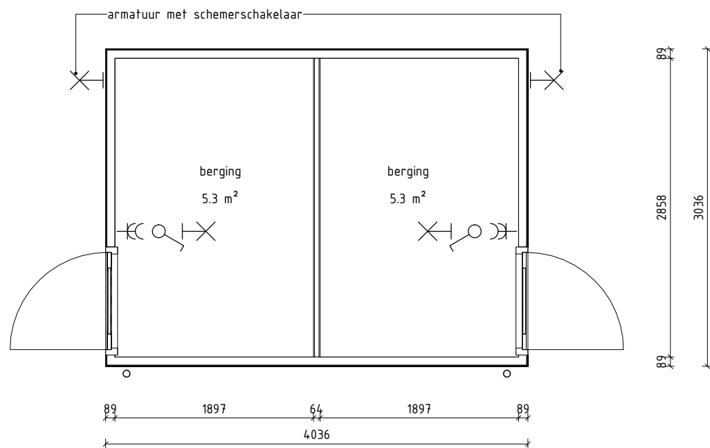
PLATTEGROND 1 : 50
