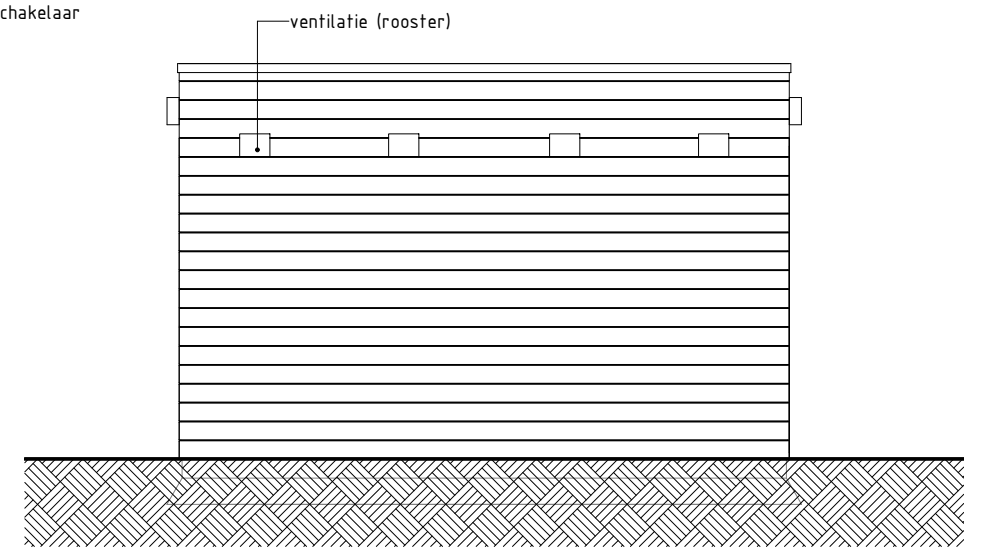
ACHTERGEVEL 1 : 50
