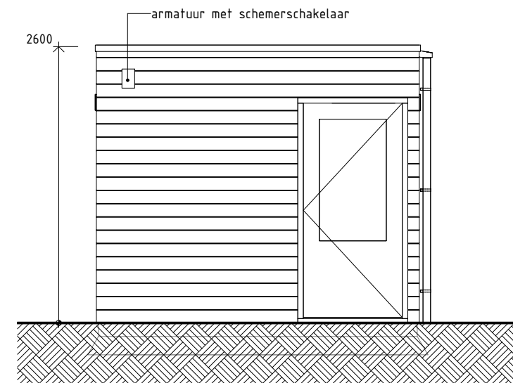
ZIJGEVEL LINKS 1 : 50
