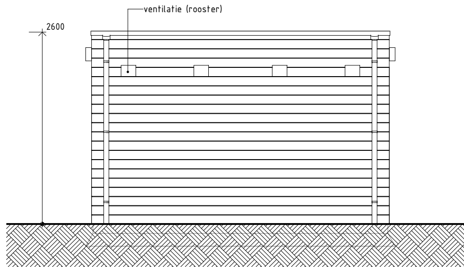
VOORGEVEL (vanuit de woning gezien) 1 : 50
