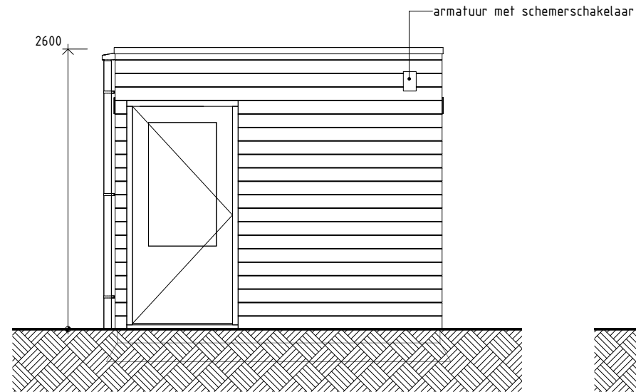
ZIJGEVEL RECHTS 1 : 50
